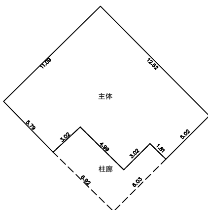
第1层平面图
