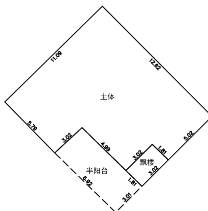
第2层平面图
