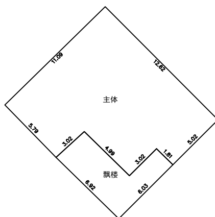
第3层平面图
