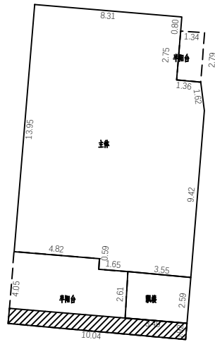
2层平面图
