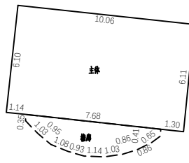
3层平面图
