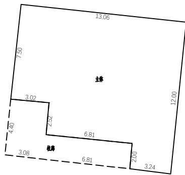
1层平面图
